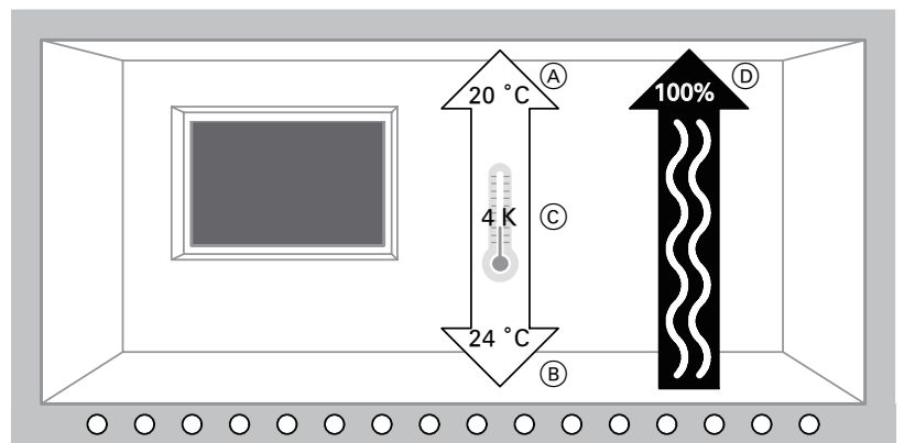
大面积辐射散热，优化的热量分布
