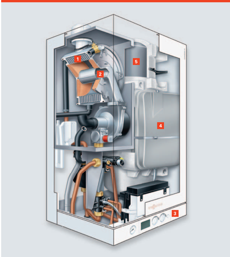
Vitodens 111-W (B1LA)
